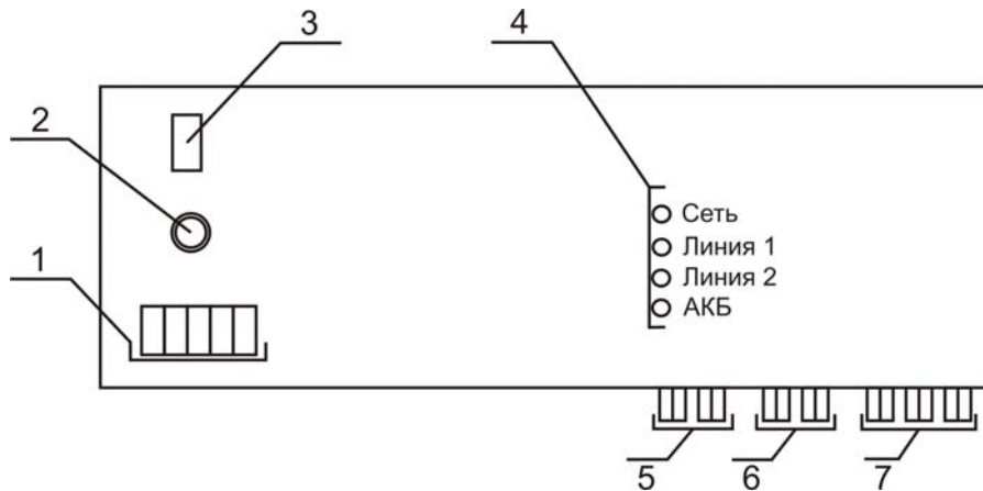
Рис. 2 Шасси преобразователя
